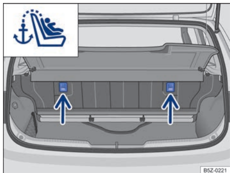
Fig. 37 Olhais de retenção para o cinto de fixação superior no lado de trás do banco traseiro.
