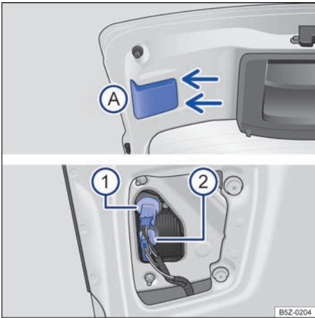
Fig. 158 Lanterna traseira: (A) desinstalar a cobertura e ① e ② desinstalar as lâmpadas.
