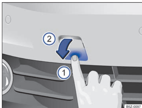
Fig. 169 No para-choque dianteiro à direita: soltar e remover a cobertura.
