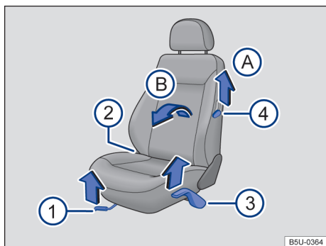
Fig. 56 Comandos do banco dianteiro esquerdo.
