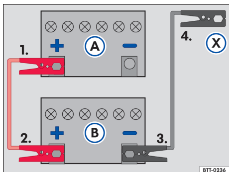
Fig. 124 Esquema para a conexão dos cabos auxiliares de partida: bateria do veículo descarregada (A) e bateria do veículo fornecedora de corrente (B).
