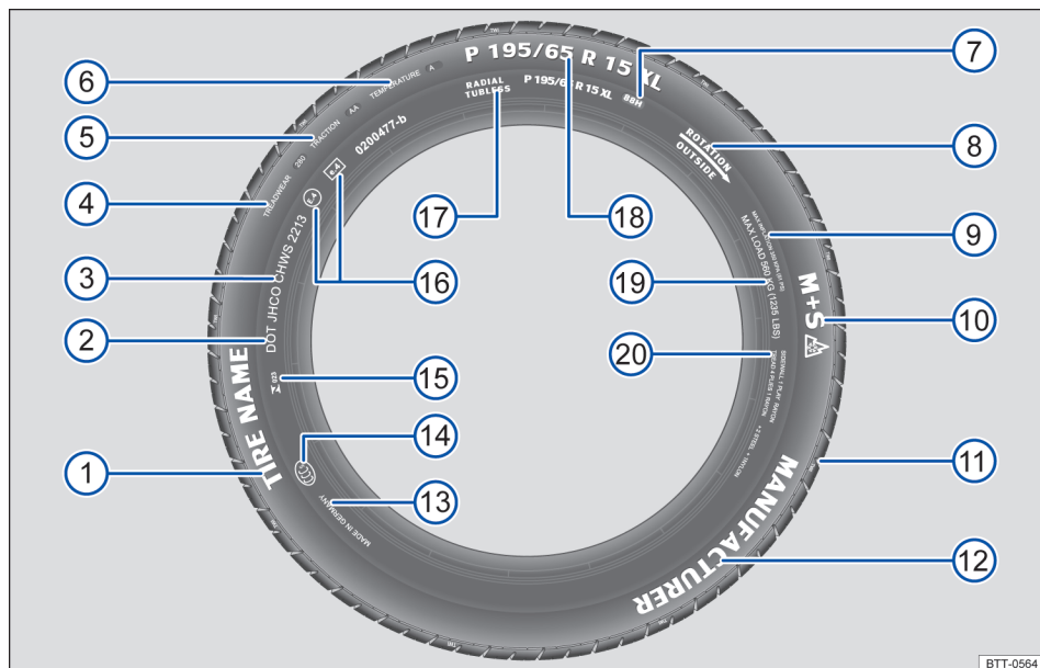
Fig. 140 Inscrição dos pneus internacional (exemplo).
