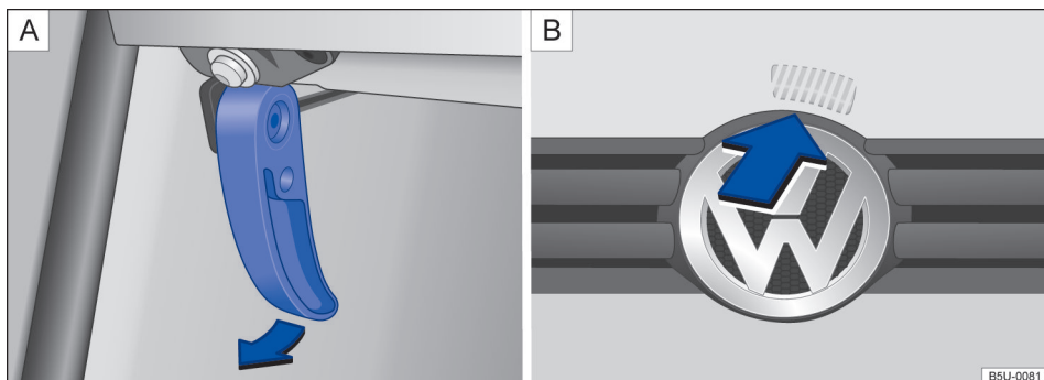
Fig. 125 A Alavanca de destravamento da tampa do compartimento do motor na área para os pés do lado do condutor. B Alavanca de destravamento na parte interna da tampa do compartimento do motor.
