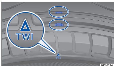
Fig. 138 Perfil do pneu: indicadores de desgaste.
