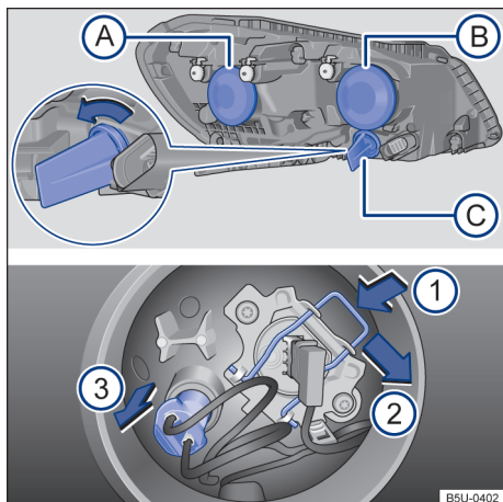
Fig. 110 No compartimento do motor: vista traseira do farol dianteiro com cobertura de borracha (lado esquerdo da ilustração) - A farol baixo, B farol alto e luz de posição, e C indicador de direção. Vista traseira do farol dianteiro sem a cobertura de borracha (lado direito da ilustração): 1 mola de travamento da lâmpada incandescente do farol e 2 luz de posição.
