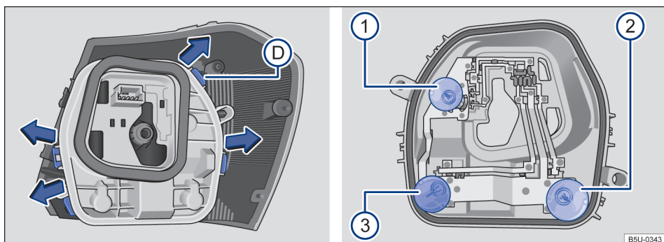
Fig. 114 Lanterna traseira: (D) desinstalar o suporte das lâmpadas e 1, 2 e 3 desinstalar as lâmpadas.
