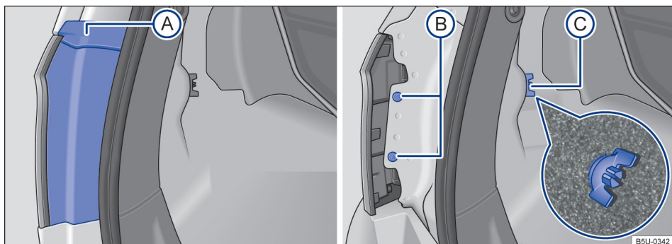
Fig. 113 No compartimento de bagagem: (A) desinstalar cobertura, (B) retirar os dois parafusos de fixação e (C) retirar o parafuso borboleta (lupa).
