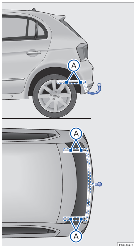
Fig. 101 Pontos de fixação para instalar um dispositivo de reboque posteriormente.
