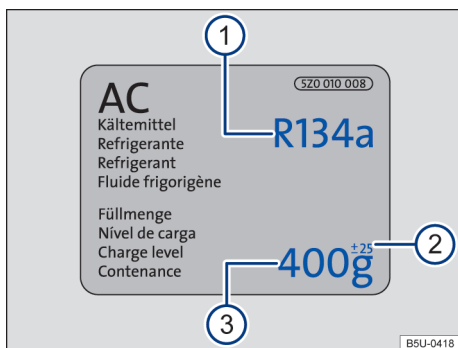
Fig. 153 Informações do ar-condicionado.
