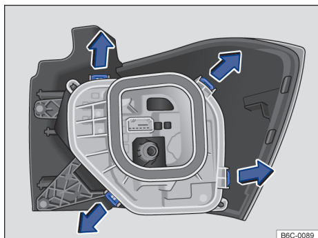
Fig. 136 Lanterna traseira: desinstalar o suporte das lâmpadas
