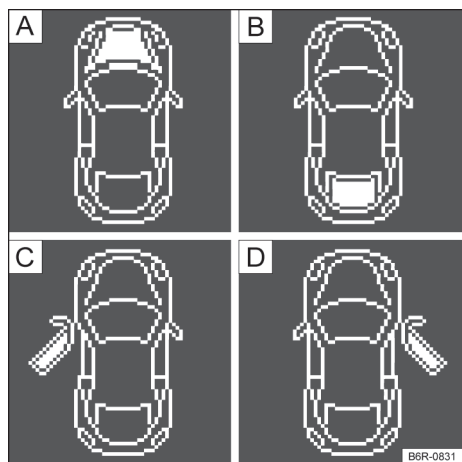
Fig. 14 No display do instrumento combinado: indicadores de status da tampa do compartimento do motor, da tampa do compartimento de bagagem e das portas.
