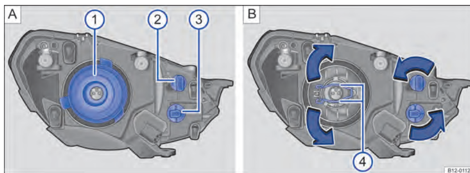
Fig. 106 No compartimento do motor: vista traseira do farol dianteiro esquerdo com cobertura de borracha: ① farol baixo e farol alto, ② luz de posição e/ou luz de condução diurna, ③ indicadores de direção e trava de proteção ④.
