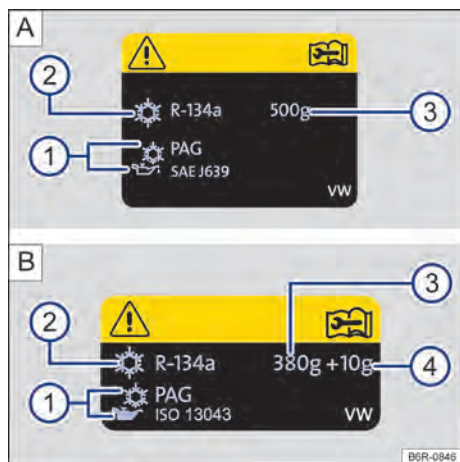
Fig. 151 (A): Informações do ar-condicionado - motor TSI. (B) Informações do ar-condicionado - motor MPI.
