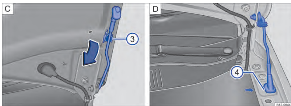
Fig. 123 C: haste de sustentação da tampa do compartimento do motor. D: tampa do motor protegida com a haste de sustentação da tampa.
