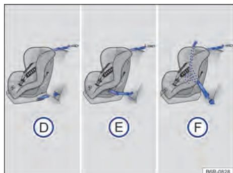
Fig. 36 No banco traseiro: as figuras (D) e (E) mostram o princípio da fixação do sistema de retenção para crianças nos olhais de retenção inferiores e com o cinto de fixação superior. A figura (F) mostra a fixação do sistema de retenção para crianças com o cinto de segurança do veículo e com o cinto de fixação superior.
