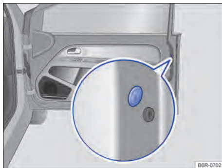
Fig. 54 Na parte dianteira da porta do passageiro dianteiro: travamento de emergência, coberto por uma vedação de borracha.
