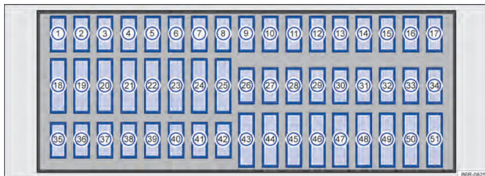
Fig. 115 Caixa de fusíveis.
