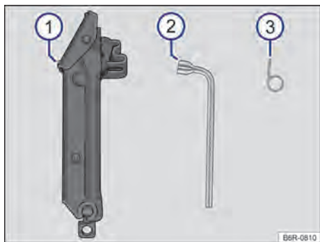
Fig. 102 Representação esquemática: componentes das ferramentas de bordo.
