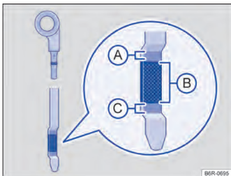
Fig. 125 Varetas de medição do óleo com marcas de nível do óleo do motor.
