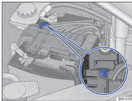
Fig. 131 No compartimento do motor: exemplo de posição do visor no lado superior da bateria do veículo.
