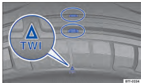
Fig. 135 Perfil do pneu: indicadores de desgaste.
