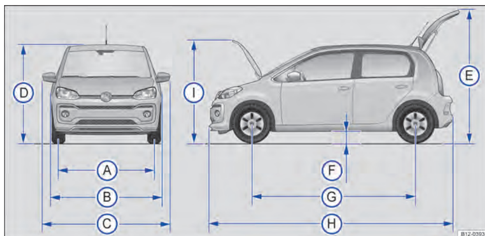
Fig. 152 Dimensões.
