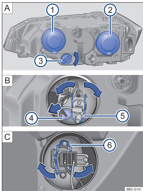
Fig. 129 No compartimento do motor: ① farol alto e luz de posição, ② farol baixo e ③ indicador de direção.
