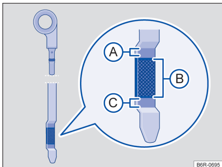
Fig. 149 Varetas de medição do óleo com marcas de nível do óleo do motor.
