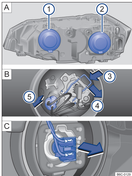
Fig. 127 No compartimento do motor: ① farol alto e luz de posição e ② farol baixo.
