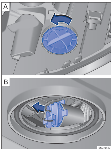
Fig. 128 Farol dianteiro, por baixo: cobertura do indicador de direção.
