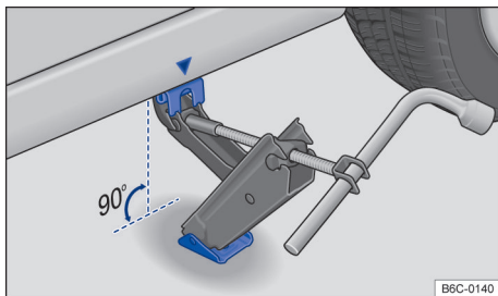
Fig. 166 Pontos de apoio do macaco e macaco posicionado no lado esquerdo traseiro do veículo.
