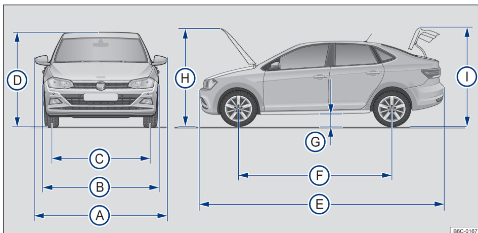
Fig. 173 Dimensões.
